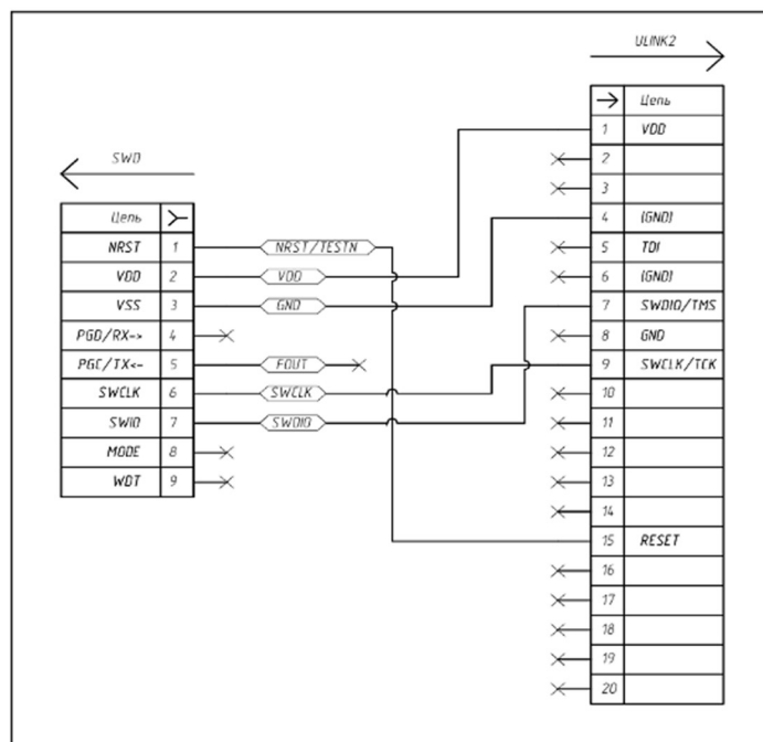
Рисунок 1 – Схема подключения программатора к плате RS-485-модуля
