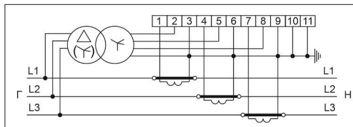
Рисунок Б.3 – Схема включения счетчиков в корпусах D37 и W37 трансформаторного включения через три трансформатора тока
