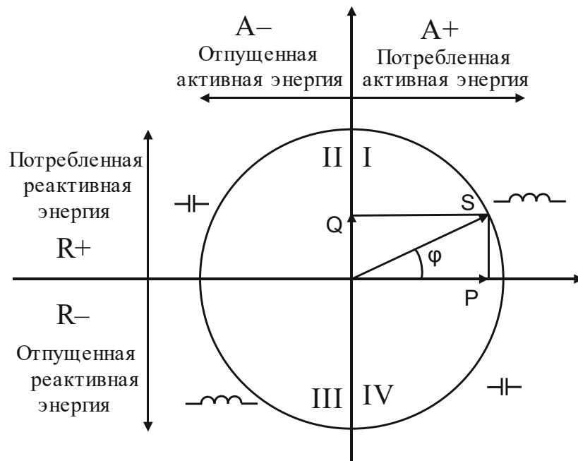
Рисунок 2.5 – Диаграмма распределения активной и реактивной мощности (энергии) по квадрантам
