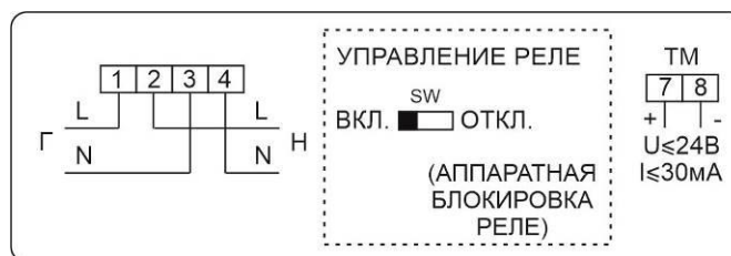
Рисунок Б.36 – Схема включения счетчиков в корпусах W9 с одним дискретным выходом, настроенным как телеметрический выход (ТМ) и аппаратной блокировкой встроенного реле управления нагрузкой (с помощью микропереключателя)
