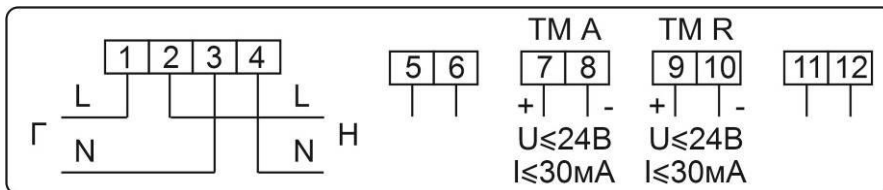
Рисунок Б.21 – Схема включения счетчиков в корпусах W3 с двумя (независимыми) дискретными выходами, настроенными как телеметрический выход активной энергии (TM A) и реактивной энергии (TM R)
