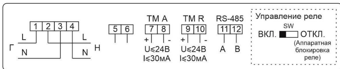
Рисунок Б.26 – Схема включения счетчиков в корпусах W3 с интерфейсом RS-485, с двумя (независимыми) дискретными выходами, настроенными как телеметрический выход активной энергии (TM A) и реактивной энергии (TM R) и аппаратной блокировкой встроенного реле управления нагрузкой (с помощью микропереключателя)
