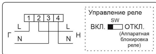
Рисунок Б.42 – Схема включения счетчиков в корпусах SP2 и аппаратной блокировкой встроенного реле управления нагрузкой (с помощью микропереключателя)
