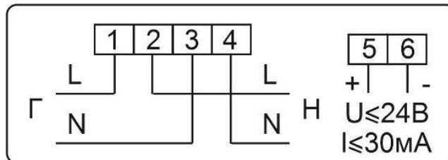
Рисунок Б.28 – Схема включения счетчиков в корпусах W6, W6b, W9 с одним дискретным выходом
