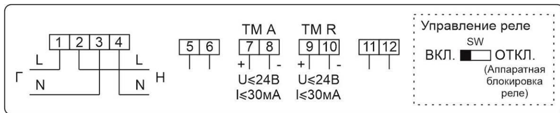
Рисунок Б.24 – Схема включения счетчиков в корпусах W3 с двумя (независимыми) дискретными выходами, настроенными как телеметрический выход активной энергии (TM A) и реактивной энергии (TM R) и аппаратной блокировкой встроенного реле управления нагрузкой (с помощью микропереключателя)
