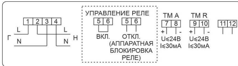
Рисунок Б.23 – Схема включения счетчиков в корпусах W3 с двумя (независимыми) дискретными выходами, настроенными как телеметрический выход активной энергии (TM A) и реактивной энергии (TM R) и аппаратной блокировкой встроенного реле управления нагрузкой (с помощью клеммника)
