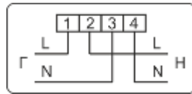
Рисунок Б.1 – Схема включения счетчиков МИРТЕК-12-АМ-W1, МИРТЕК-12-АМ-W2, МИРТЕК-12-АМ-W6, МИРТЕК-12-АМ-W6b, МИРТЕК-12-АМ-W9
