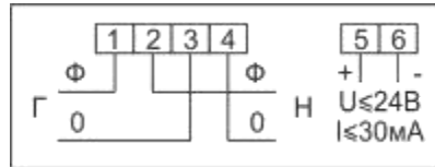
Рисунок Б.10 – Схема включения счетчиков МИРТЕК-12-АМ-SP1, МИРТЕК-12-АМ-SP3
