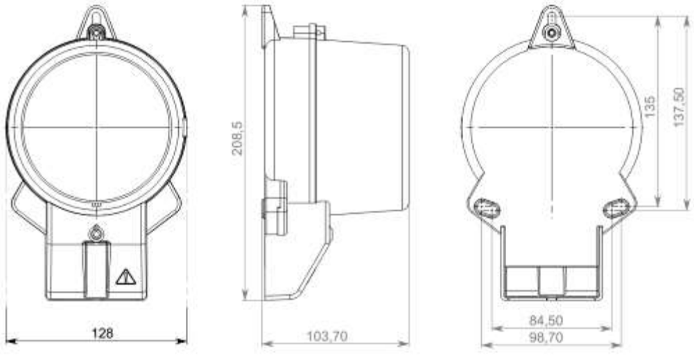
Рисунок В.4 – Тип корпуса W6
