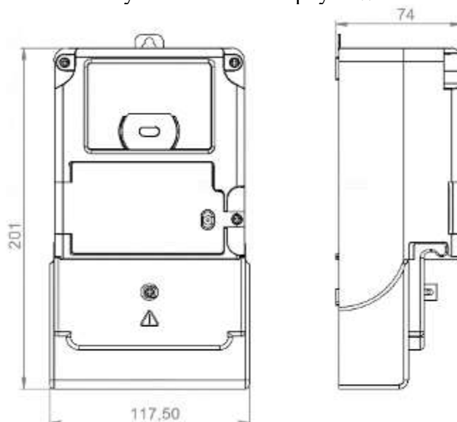
Рисунок В.3 – Тип корпуса W3
