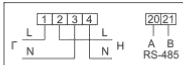
Рисунок Б.4 – Схема включения счетчиков МИРТЕК-12-АМ-W2-xx-RS485
