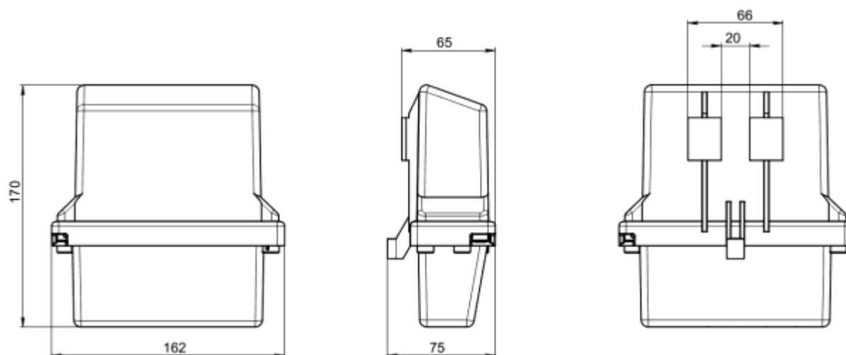
Рисунок В.12 – Тип корпуса «SP3»
