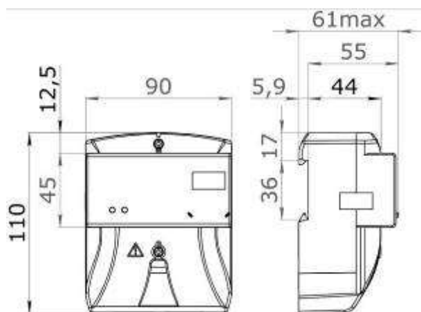
Рисунок В.9 – Тип корпуса D5
