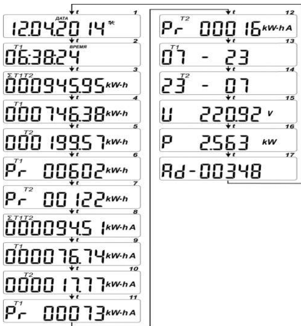
Рисунок 3.3 – Режимы циклической индикации счётчика
