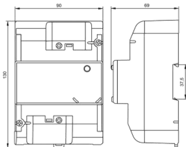
Рисунок В.7– Тип корпуса D1
