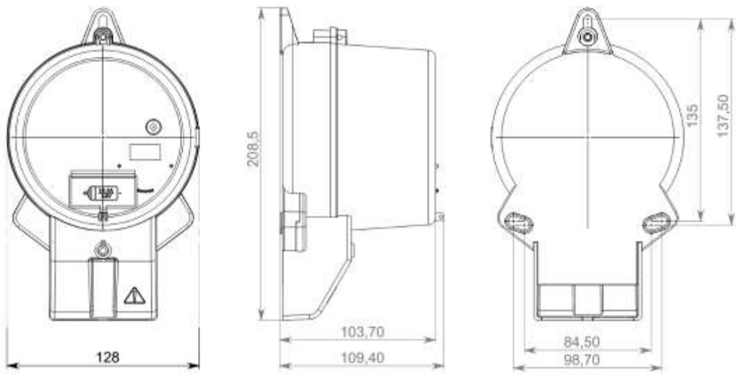
Рисунок В.5 – Тип корпуса W6b
