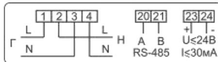
Рисунок Б.5 – Схема включения счетчиков МИРТЕК-12-АМ-W2-xx-RS485-Q1
