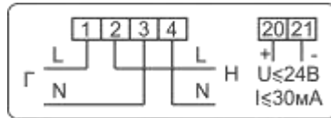
Рисунок Б.2 – Схема включения счетчиков МИРТЕК-12-АМ-W2-xx-Q1
