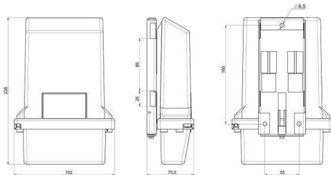
Рисунок В.10 – Тип корпуса «SP1»
