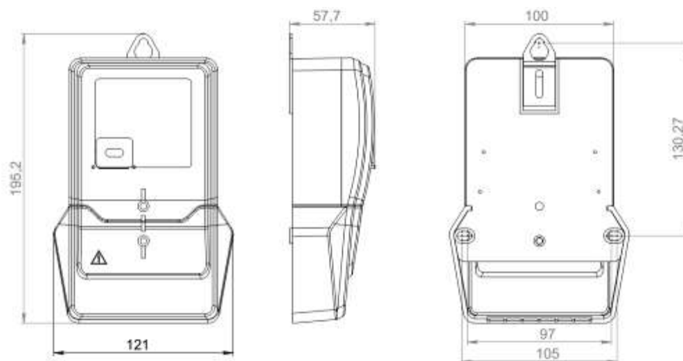
Рисунок В.1 – Тип корпуса W1
