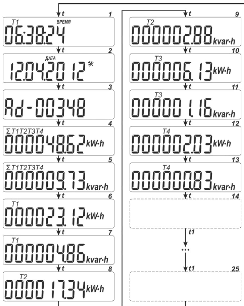
Рисунок 3.4 – Режимы циклической индикации счетчика
