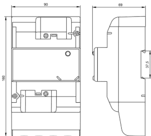
Рисунок В.8 – Тип корпуса D4
