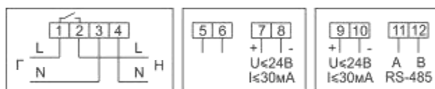
Рисунок Б.8 – Схема включения счетчиков МИРТЕК-12-АМ-W3-A1R1-230-5-60A-S-RS485-xx-KLMOQ2V3
