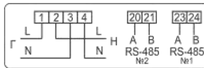
Рисунок Б.3 – Схема включения счетчиков МИРТЕК-12-АМ-W2-xx-RS485-RS485-xx
