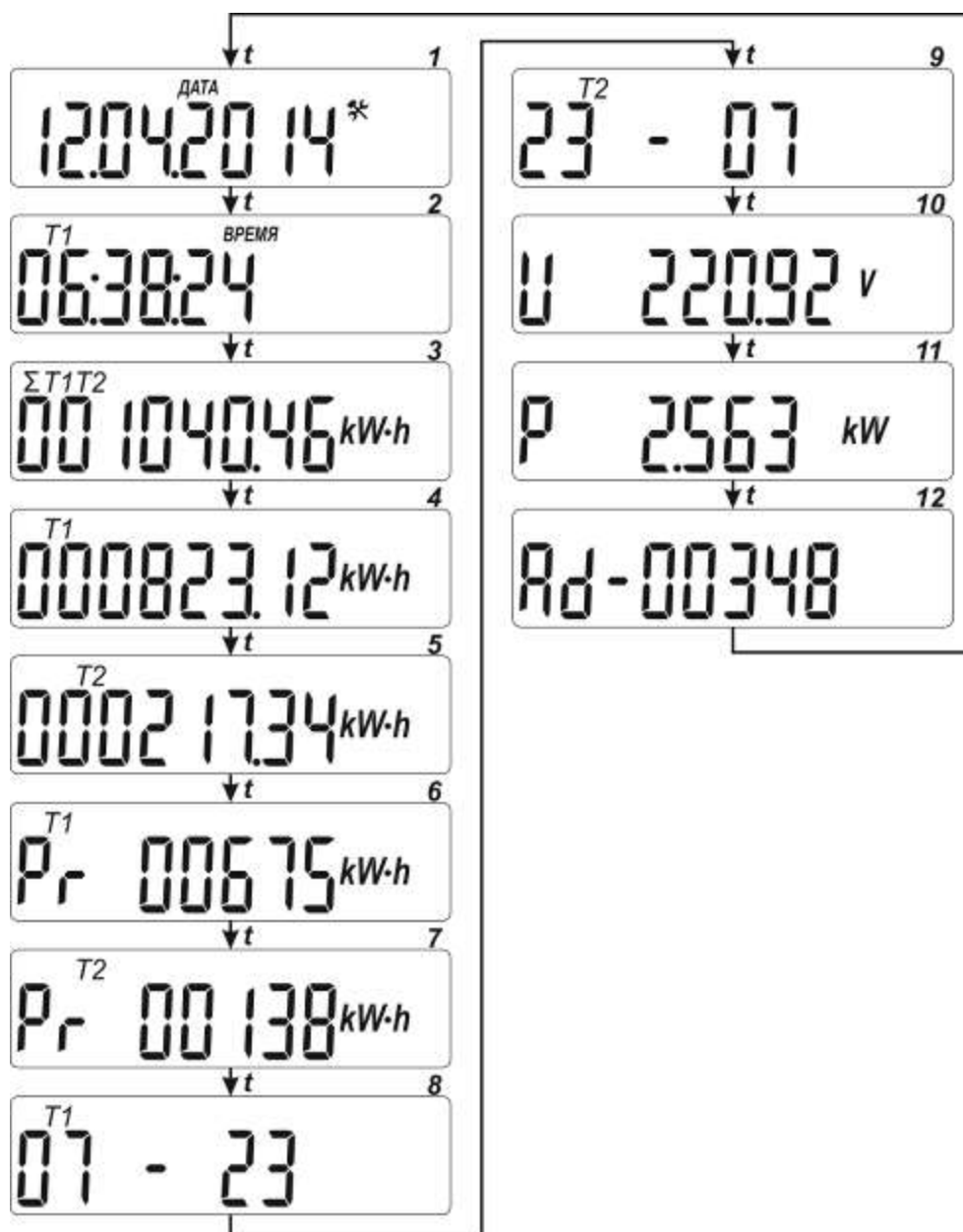
Рисунок 3.2 – Режимы циклической индикации счётчика
