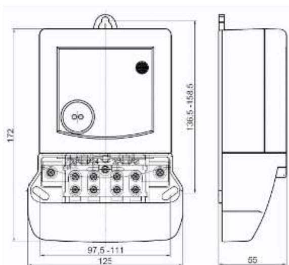
Рисунок В.2 – Тип корпуса W2
