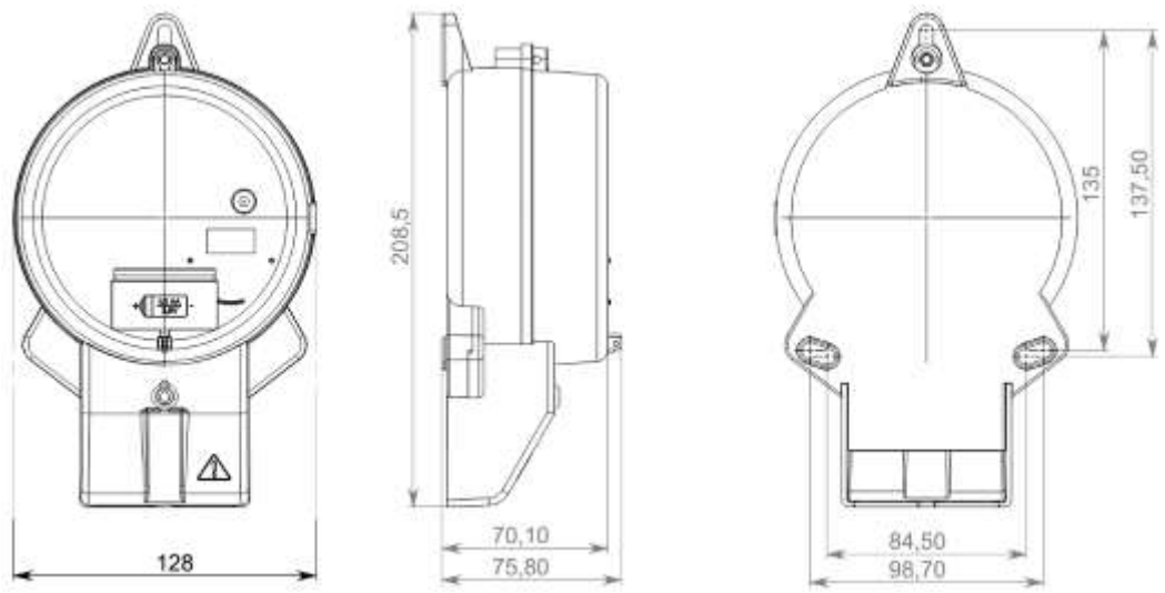
Рисунок В.6 – Тип корпуса W9
