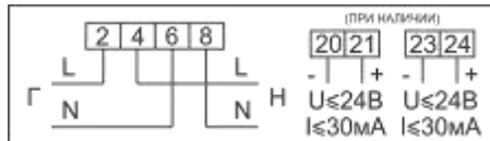
Рисунок Б.6 – Схема включения счетчиков МИРТЕК-12-АМ-D1, МИРТЕК-12-АМ-D4
