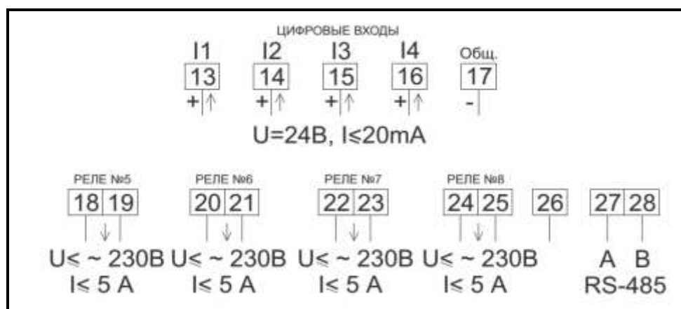
Рисунок Б.15 – Подключение сигнальных цепей счетчика в корпусе W32 с интерфейсами RS485-I4Q4Z
