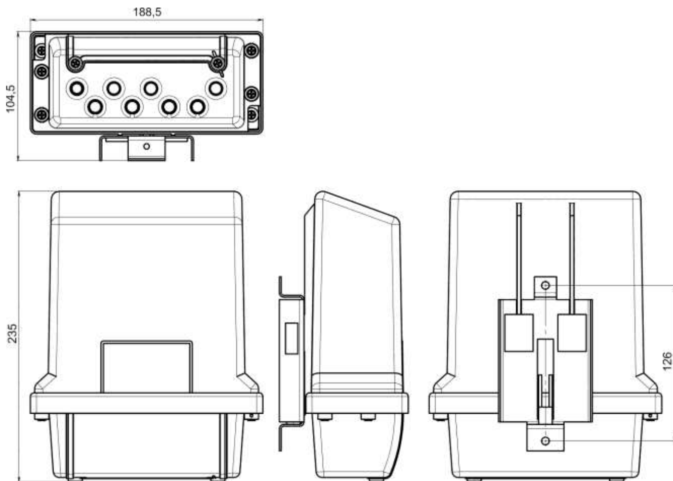
Рисунок В.8 – Тип корпуса SP31
