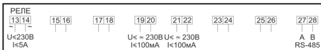
Рисунок Б.12 – Подключение сигнальных цепей счетчика в корпусе W32 с интерфейсами RS485-Q3
