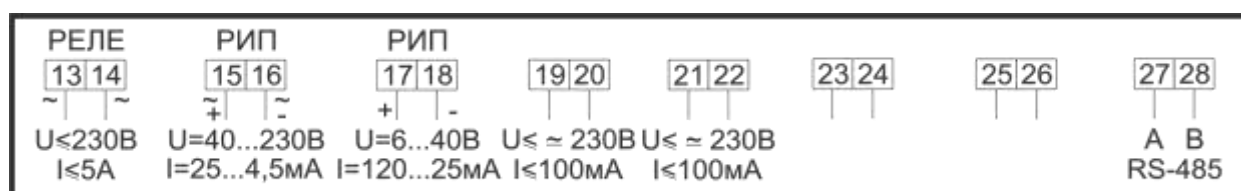
Рисунок Б.14 – Подключение сигнальных цепей счетчика в корпусе W32 с интерфейсами RS485-Q3Z
