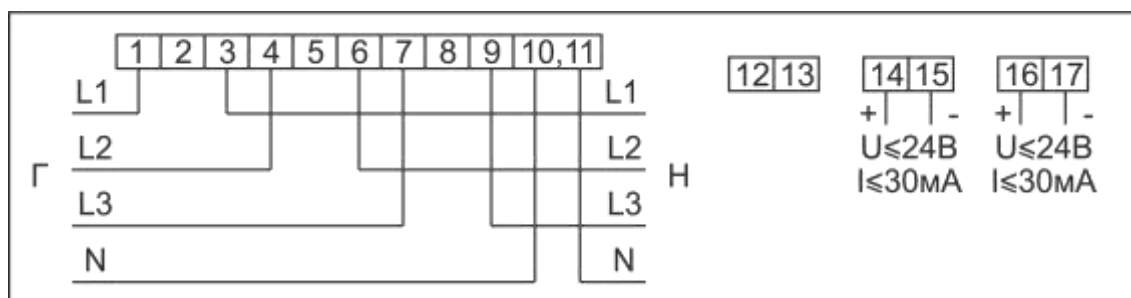
Рисунок Б.1 – Схема включения счетчиков в корпусах W31 и D33 непосредственно-го включения со встроенным радиointерфейсом с двумя дискретными выходами
