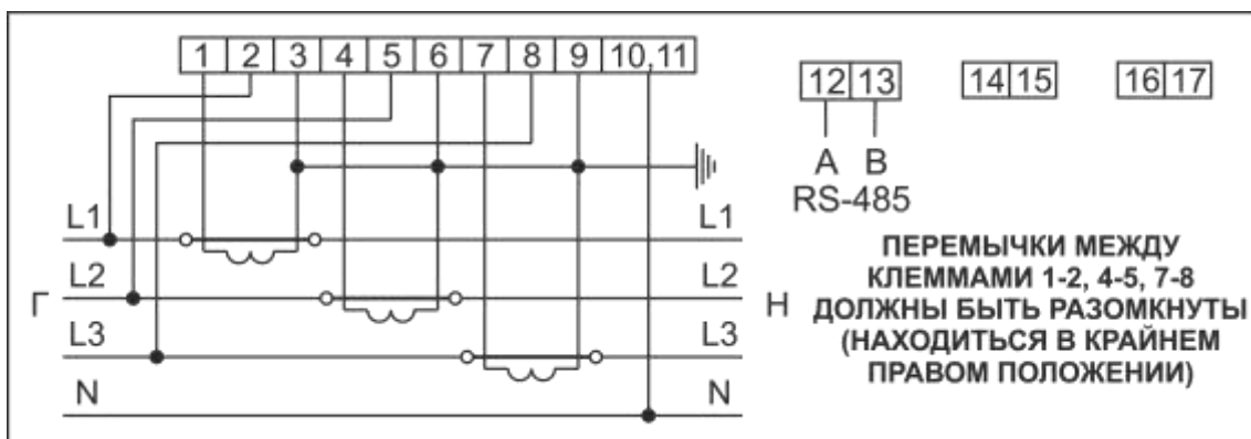
Рисунок Б.5 – Схемы включения счетчиков в корпусах W31 и D33 через трансформатор тока со встроенным модулем интерфейса RS485
