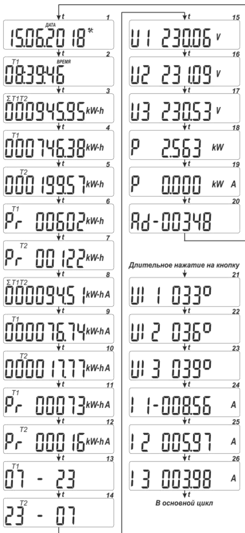
Рисунок 3.7 – Режимы циклической индикации счётчика
