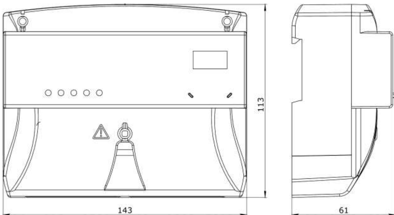
Рисунок В.7 – Тип корпуса D35
