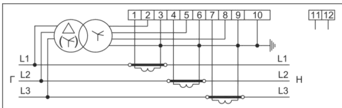
Рисунок Б.9 – Схема включения счетчиков в корпусе W32 через трансформаторы тока и трансформаторы напряжения
