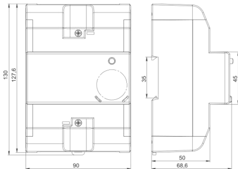
Рисунок В.4 – Тип корпуса D31
