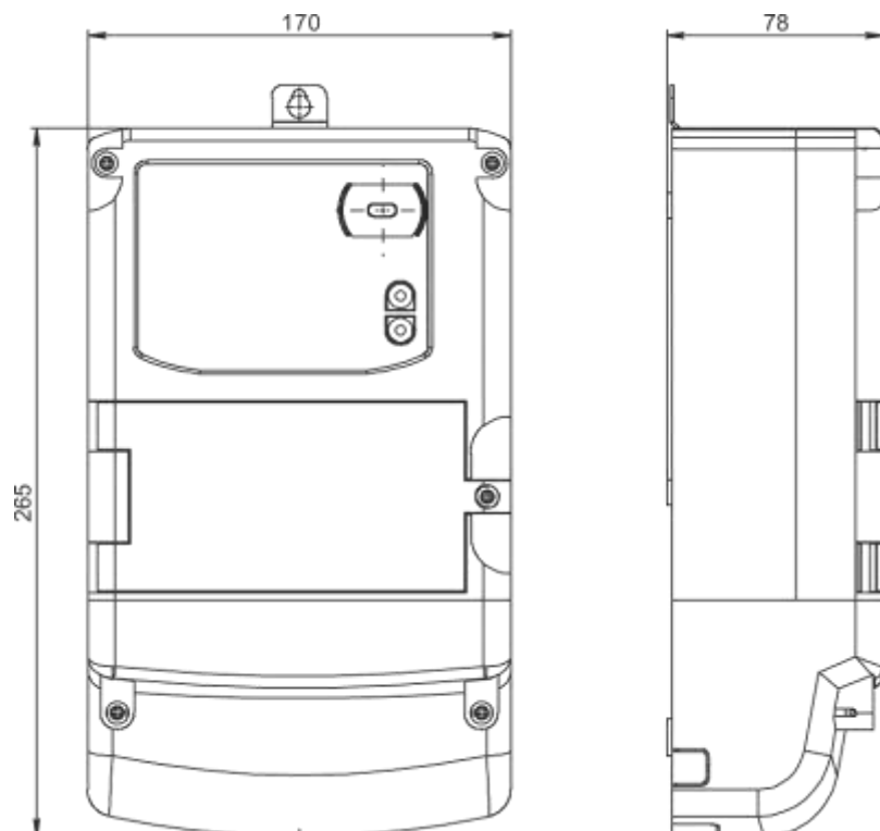
Рисунок В.3 – Тип корпуса W33
