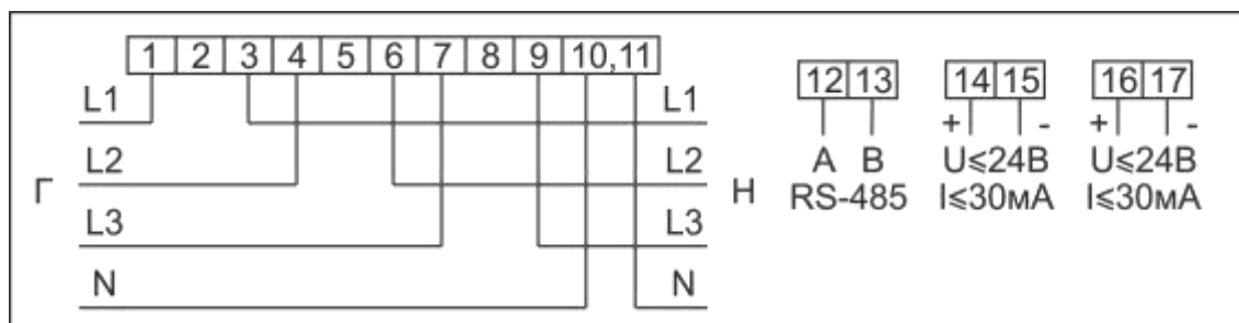
Рисунок Б.3 – Схема включения счетчиков в корпусах W31 и D33 непосредственно-го включения со встроенным модулем интерфейса RS485 с двумя дискретными вы-ходами
