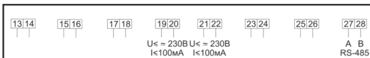
Рисунок Б.11 – Подключение сигнальных цепей счетчика в корпусе W32 с интерфейсами RS485-Q2
