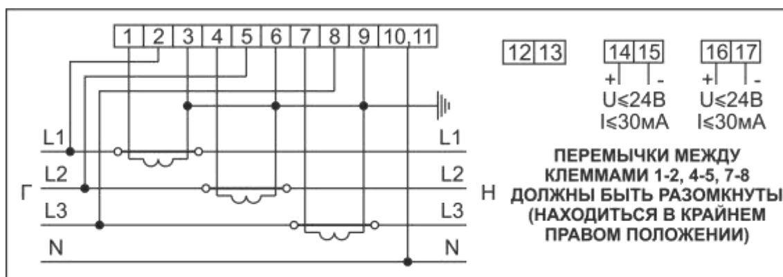
Рисунок Б.4 – Схемы включения счетчиков в корпусах W31 и D33 через трансфор-матор тока со встроенным радиointерфейсом с двумя дискретными выходами
