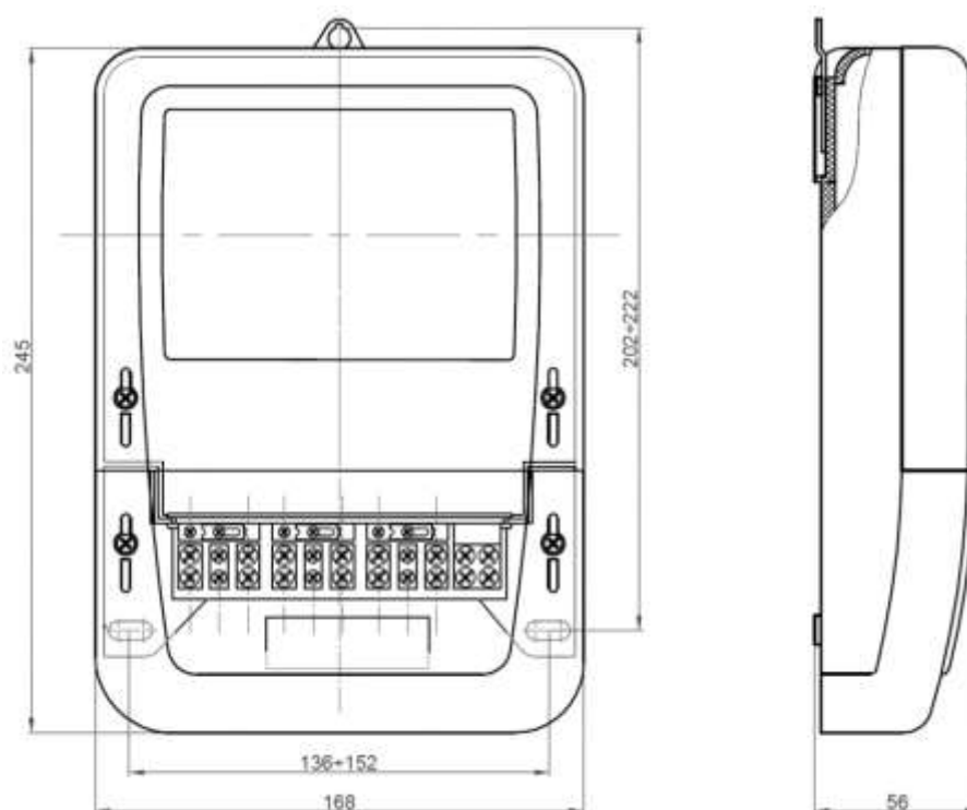
Рисунок В.1 – Тип корпуса W31
