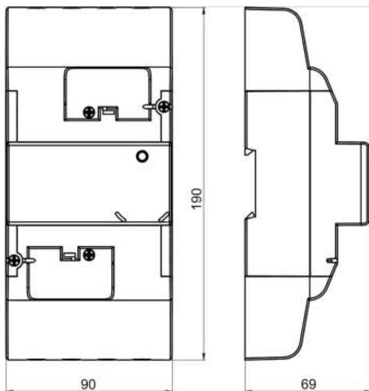
Рисунок В.6 – Тип корпуса D34
