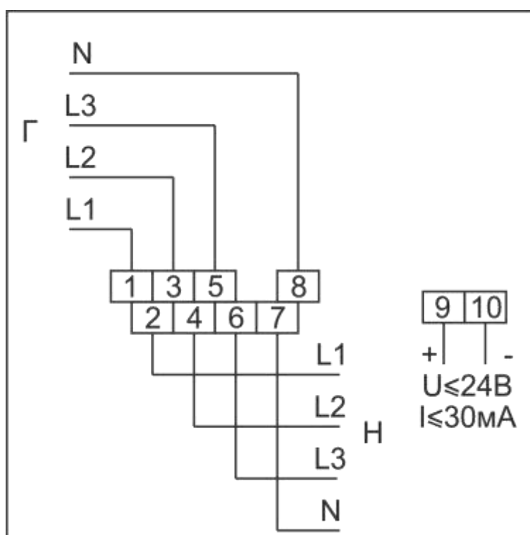
Рисунок Б.7 – Схема включения счетчиков в корпусе SP31
