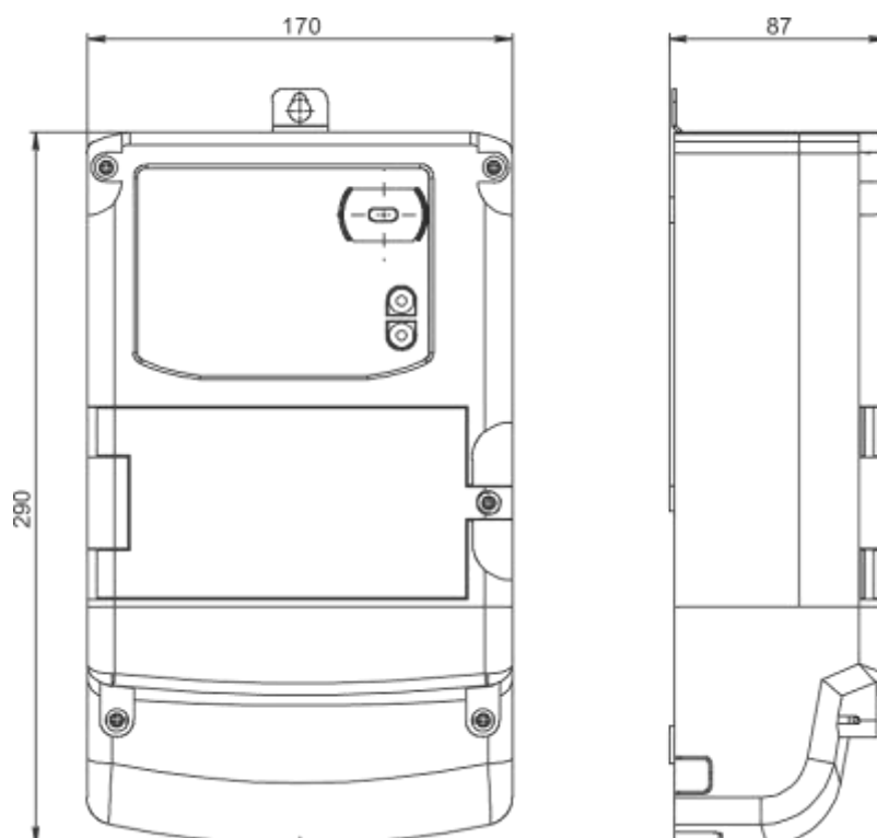
Рисунок В.2 – Тип корпуса W32
