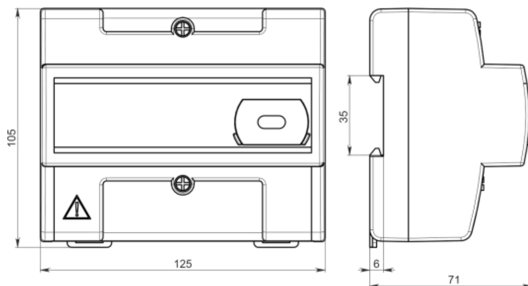
Рисунок В.5 – Тип корпуса D33
