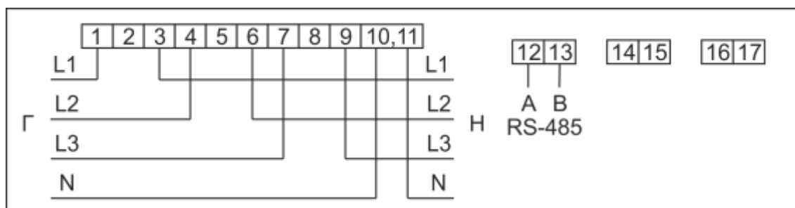
Рисунок Б.2 – Схема включения счетчиков в корпусах W31 и D33 непосредственно-го включения со встроенным модулем интерфейса RS485
