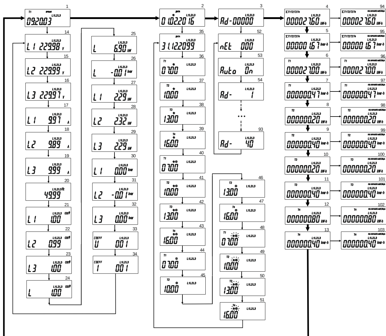
Рисунок 3.5 - Режимы циклической индикации для двунаправленного счетчика.
