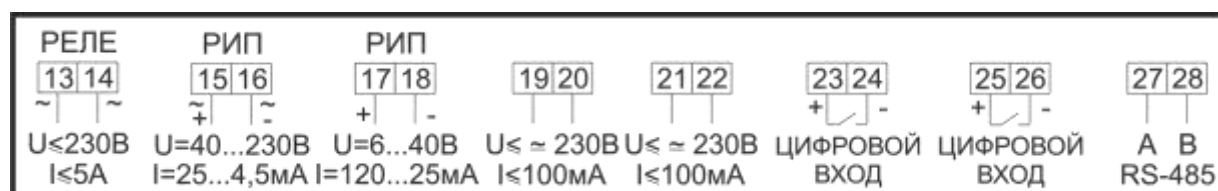
Рисунок Б.13 – Подключение сигнальных цепей счетчика в корпусе W32 с интерфейсами RS485-I2Q3Z
