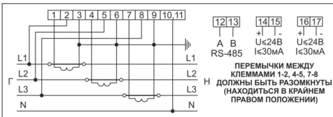
Рисунок Б.6 – Схемы включения счетчиков в корпусах W31 и D33 через трансформатор тока со встроенным модулем интерфейса RS485 с двумя дискретными выходами
