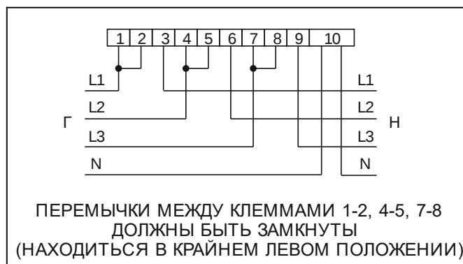
Рисунок Б.10 – Схема включения счетчиков в корпусе W32 непосредственного включения
