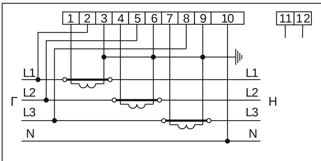
Рисунок Б.8 – Схема включения счетчиков в корпусе W32 через трансформаторы тока
