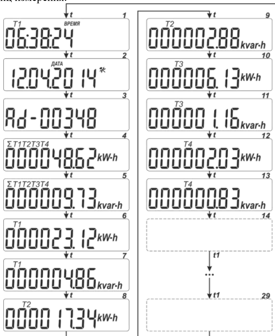
Рисунок 3.3 – Режимы циклической индикации счётчика
