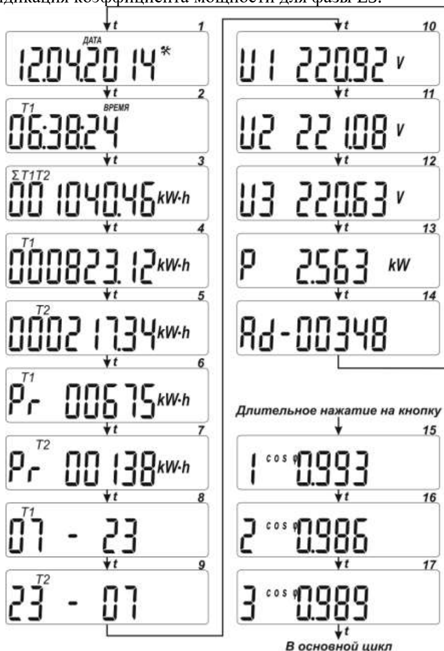
Рисунок 3.2 – Режимы циклической индикации счётчика
