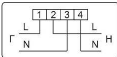
Рисунок Б.27 – Схема включения счетчиков в корпусах W6, W6b, W9
