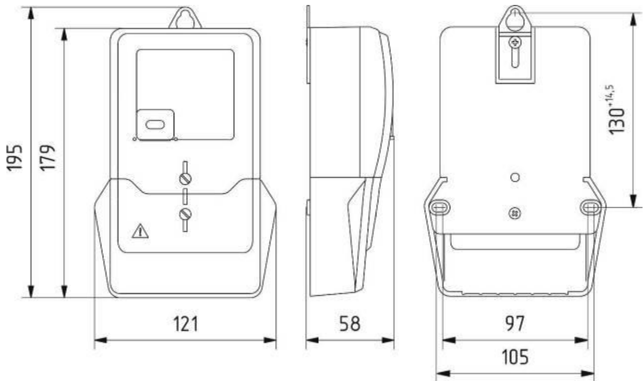
Рисунок В.1 – Тип корпуса W1
