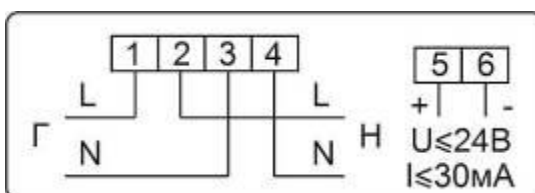
Рисунок Б.11 – Схема включения счетчиков в корпусах W1 с одним дискретным выходом
