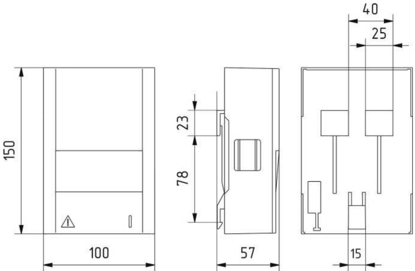
Рисунок В.11 – Тип корпуса SP2
