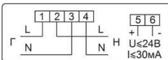
Рисунок Б.8 – Схема включения счетчиков в корпусах D5 с одним дискретным выходом
