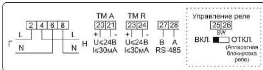
Рисунок Б.6 – Схема включения счетчиков в корпусах D1, D4 с двумя (независимыми) дискретными выходами, настроенными как телеметрический выход активной энергии (ТМ А) и реактивной энергии (ТМ R) и интерфейсом RS-485 и аппаратной блокировкой встроенного реле управления нагрузкой (с помощью микропереключателя)
