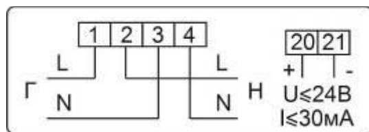
Рисунок Б.17 – Схема включения счетчиков в корпусах W2 с одним дискретным выходом
