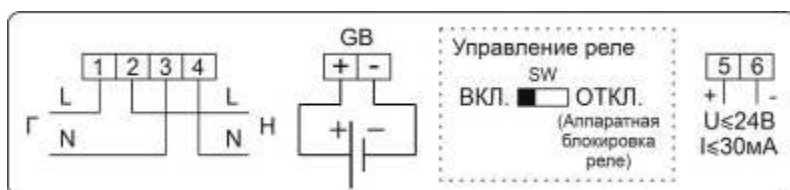
Рисунок Б.40 – Схема включения счетчиков в корпусе SP3 с одним дискретным выходом, настроенным как телеметрический выход (ТМ), разъемом для подключения дополнительной сменной батарейки (GB1) и аппаратной блокировкой встроенного реле управления нагрузкой (с помощью микропереключателя)
