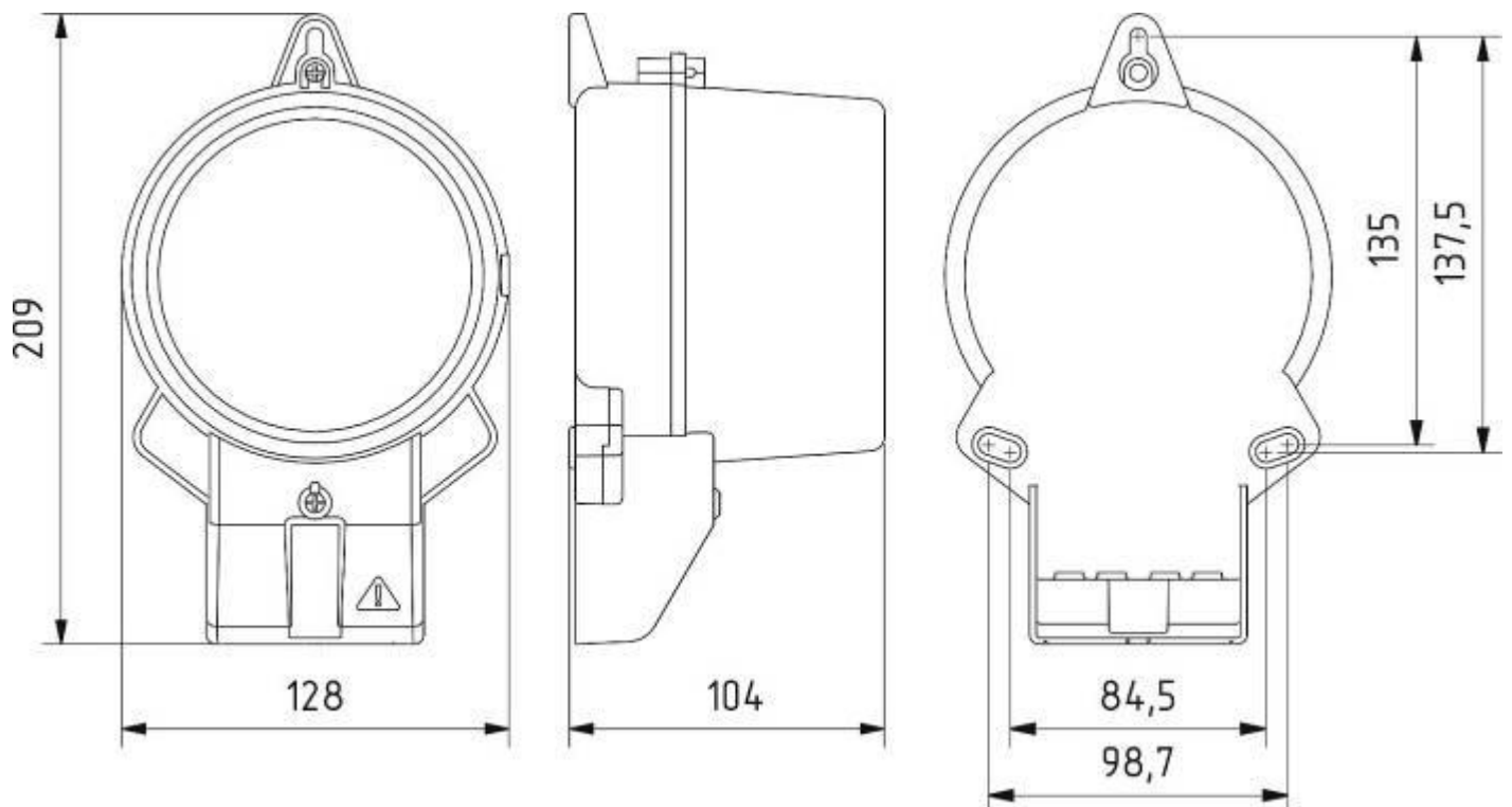
Рисунок В.4 – Тип корпуса W6
