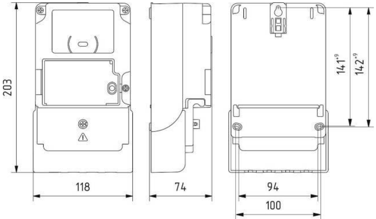
Рисунок В.3 – Тип корпуса W3
