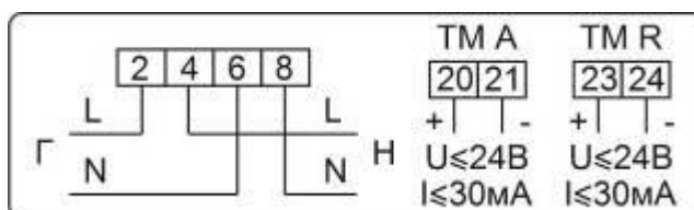
Рисунок Б.2 – Схема включения счетчиков в корпусах D1, D4 с двумя (независимыми) дискретными выходами, настроенными как телеметрический выход активной энергии (ТМ А) и реактивной энергии (ТМ R)
