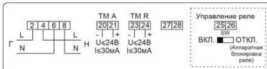
Рисунок Б.5 – Схема включения счетчиков в корпусах D1, D4 с двумя (независимыми) дискретными выходами, настроенными как телеметрический выход активной энергии (ТМ А) и реактивной энергии (ТМ R) и аппаратной блокировкой встроенного реле управления нагрузкой (с помощью микропереключателя)
