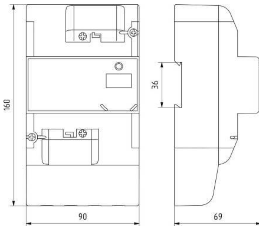
Рисунок В.8 – Тип корпуса D4
