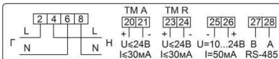
Рисунок Б.4 – Схема включения счетчиков в корпусах D1, D4 с двумя (независимыми) дискретными выходами, настроенными как телеметрический выход активной энергии (ТМ А) и реактивной энергии (ТМ R) и интерфейсом RS-485 (с внешним питанием интерфейса RS-485)
