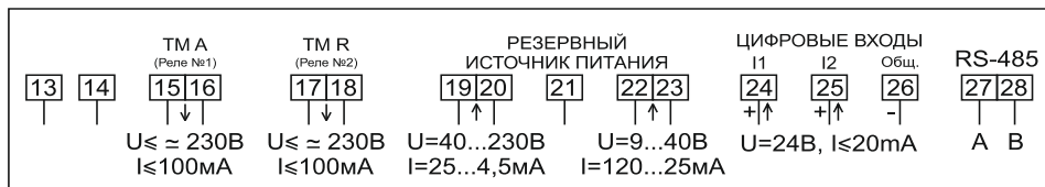
Рисунок Б.56 – Схема включения сигнальных цепей счетчиков в корпусе W32 с интерфейсом RS-485, с двумя (независимыми) дискретными выходами и с двумя дискретными входами (с одним общим проводом), с двумя входами для подключения резервного источника питания в диапазоне от 9 до 40 В и от 40 до 230 В
