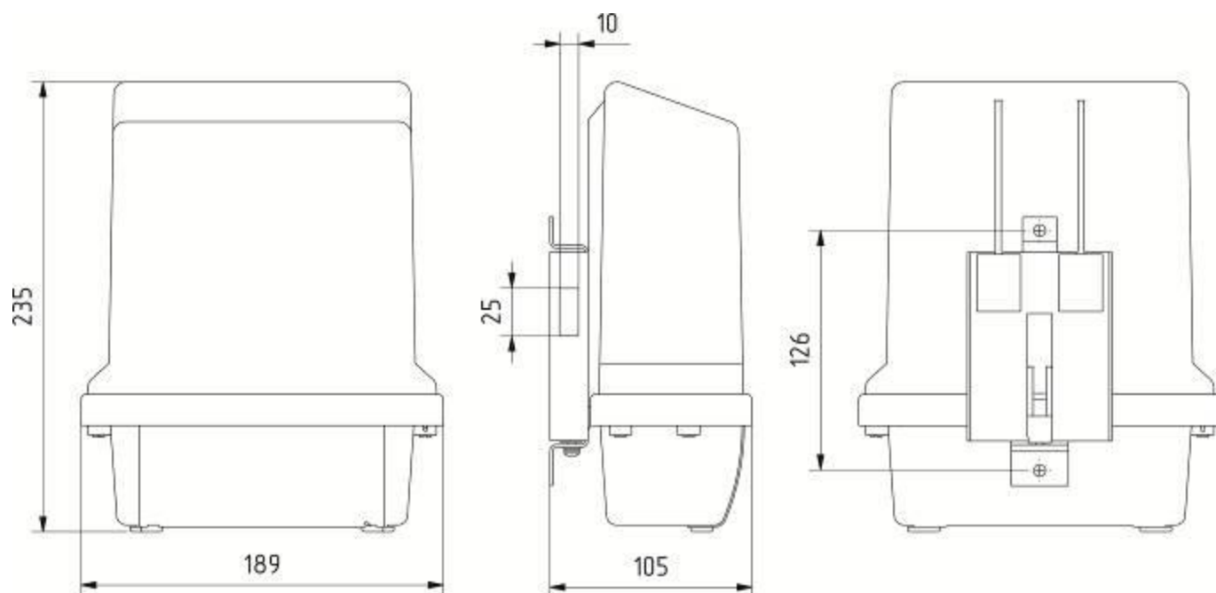
Рисунок В.9 – Тип корпуса SP31c переходной пластиной, позволяющей осуществлять монтаж на опору ВЛ-0,4 кВ и на плоскую поверхность
