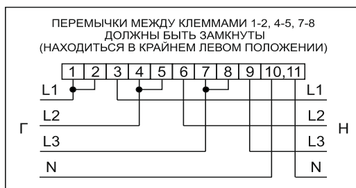
Рисунок Б.7 – Схема включения счетчиков в корпусе W31 непосредственного включения на измерительных элементах трансформатора тока
