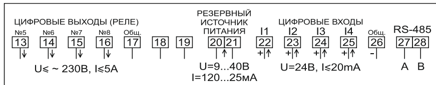
Рисунок Б.44 – Схема включения сигнальных цепей счетчиков в корпусе W32 с интерфейсом RS-485, с четырьмя дискретными выходами (с одним общим проводом) и с четырьмя дискретными входами (с одним общим проводом), с одним входом для подключения резервного источника питания в диапазоне от 9 до 40 В
