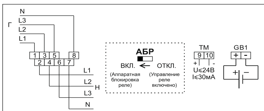
Рисунок Б.61 – Схема включения счетчиков в корпусах SP31 с одним дискретным выходом, настроенным как телеметрический выход (ТМ), разъёмом для подключения дополнительной сменной батарейки (GB1) и аппаратной блокировкой встроенного реле управления нагрузкой (с помощью микропереключателя)
